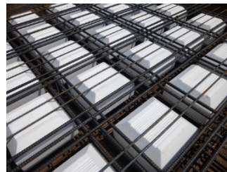
FS ボイドスラブ (H-F PCa)
