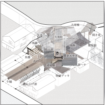
[形態検討図]
