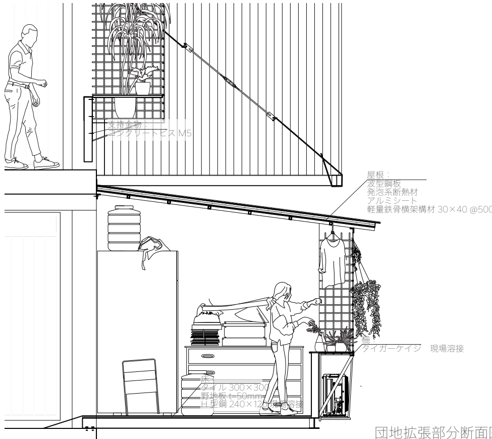
団地拡張部分断面図
